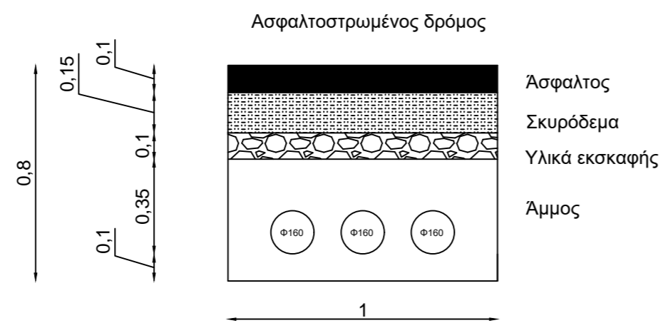
Ενδεικτικό πλάτος για τοποθέτηση τριών σωλήνων
