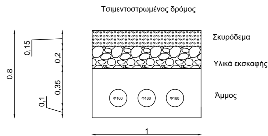
Ενδεικτικό πλάτος για τοποθέτηση τριών σωλήνων
