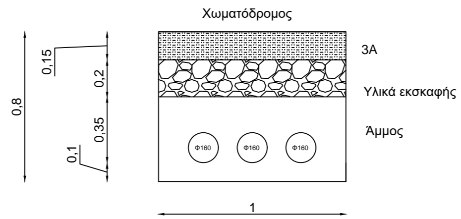
Ενδεικτικό πλάτος για τοποθέτηση τριών σωλήνων
