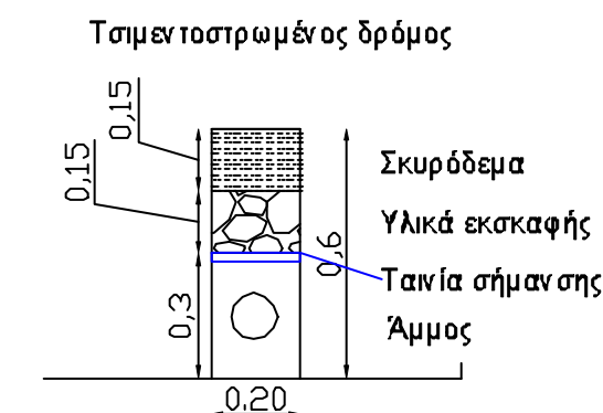
Ενδεικτικό πλάτος για εκσκαφή με τροχό (για σωλήνες Φ63 έως Φ110)
