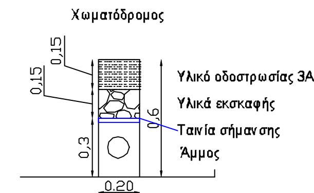
Ενδεικτικό πλάτος για εκσκαφή με τροχό (για σωλήνες Φ63 έως Φ110)
