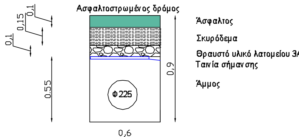
Ενδεικτικό πλάτος για αγωγό Φ225
