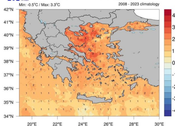
30 March 2024 SST anomaly (°C)
